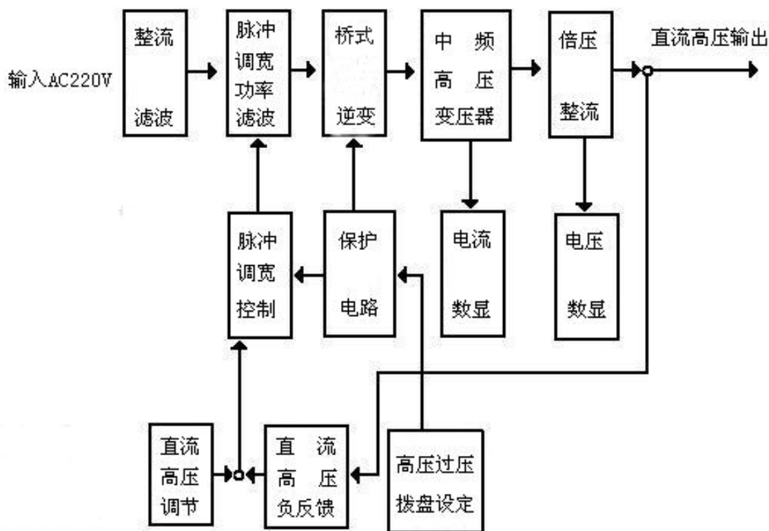
图 1 工作原理图
