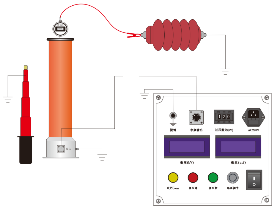
图 4 氧化锌避雷器接线图
