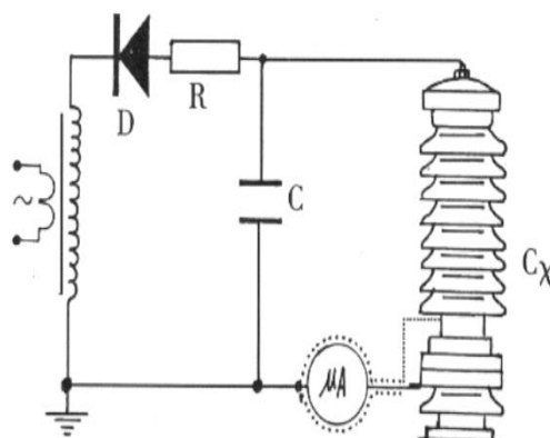
图 8 排除试品 CX 表面影响接线图
