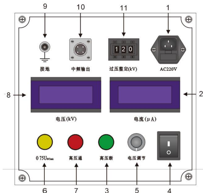
图2 面板布局图
