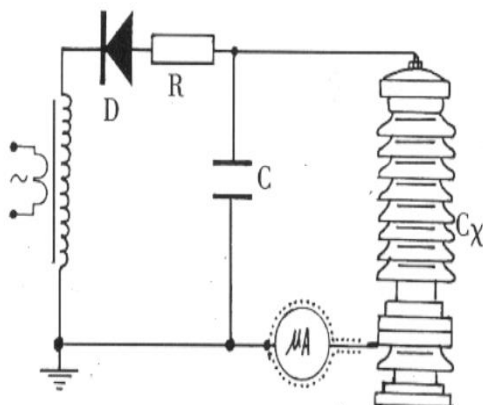
图 7 微安表接入试品 CX 底部的接线图
